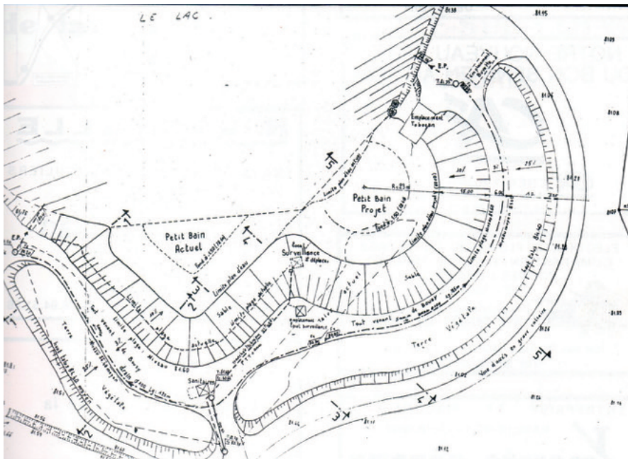
Le plan technique pour la création de la baignade
