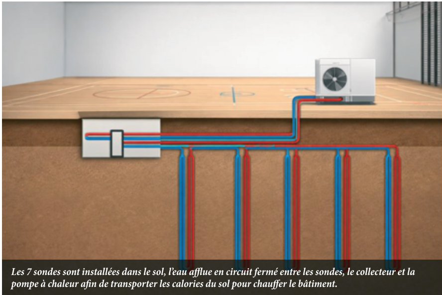
Les sondes ont été installées dans le sol grâce à un forage de tuyaux de 140 mètres de long
